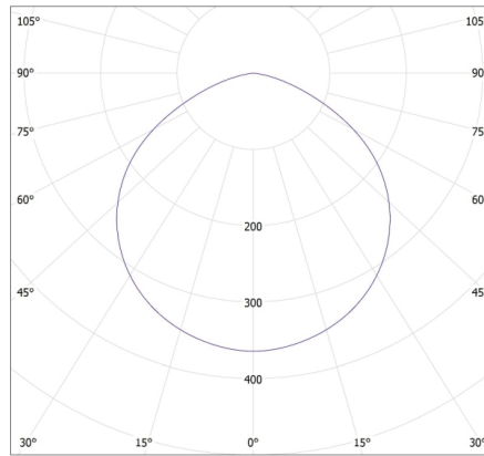
KANLUX S.A. (kat 15099) RANGO MINI R7S SMD-WW / Krzywa rozsyłu światła (biegunowo)
